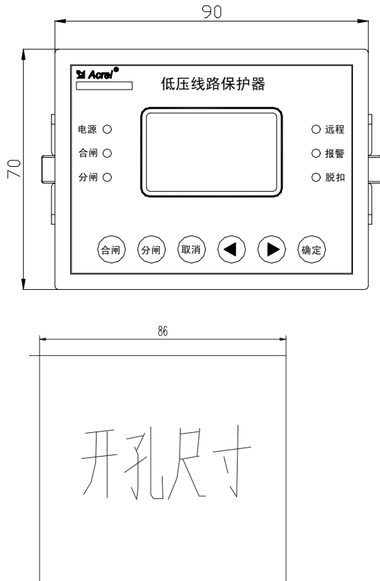
图 8 90L 显示模块外形及安装尺寸
