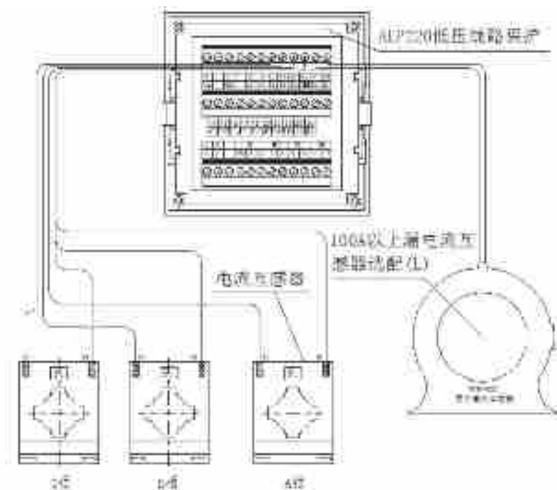
图 17 ALP220-160A、ALP220-400A 产品组成
