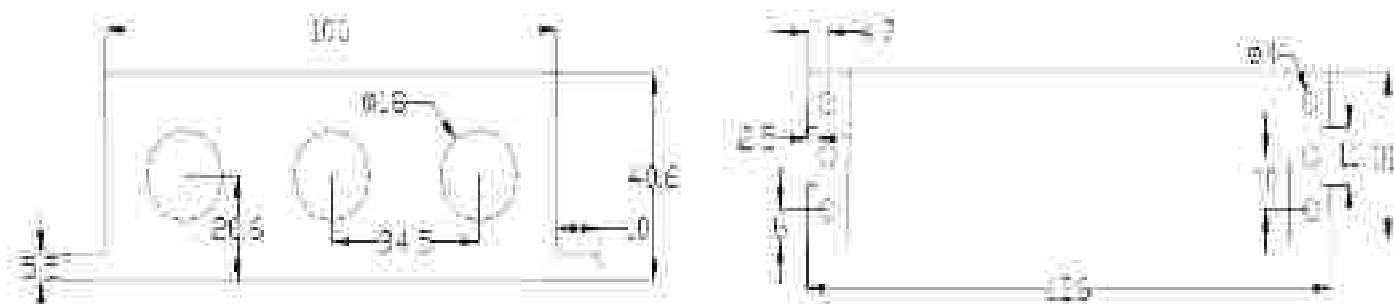
图 5 100A 及以下的电流互感器外形尺寸 Figure 5 Outline dimension of 100A and below current transformer
