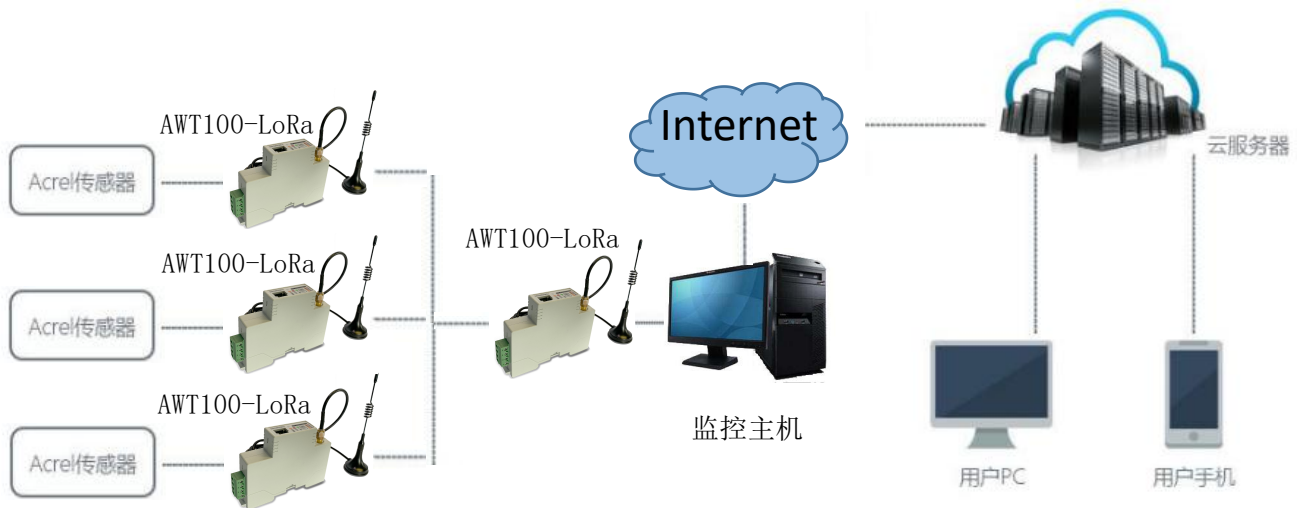
图 3 AWT100-LoRa 无线通信终端典型应用
