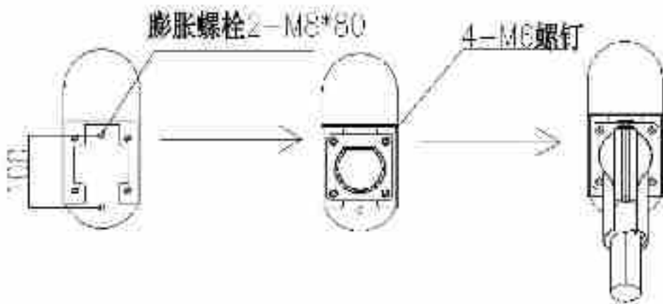
图 3-8 枪座安装顺序
