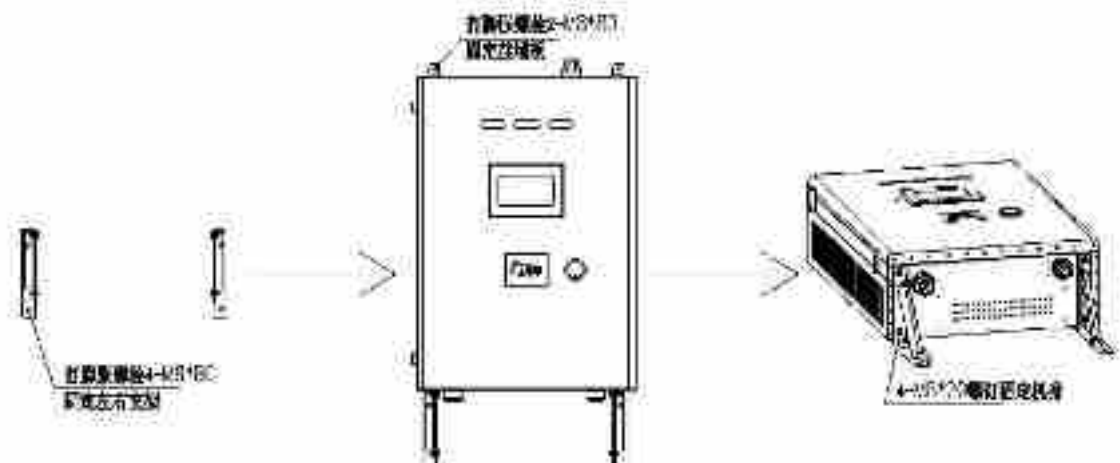
图 3-7 充电机安装顺序
