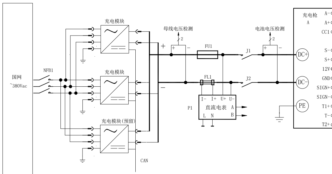
图 2-5 充电机原理框图
