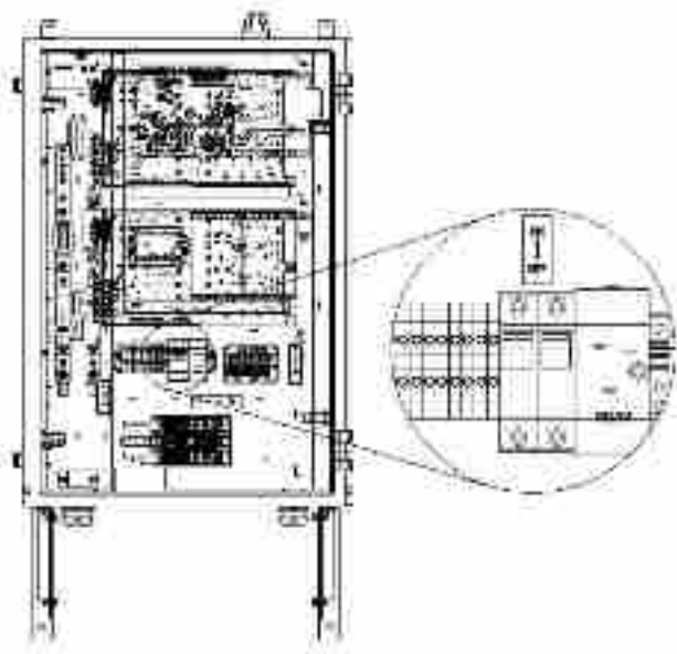
图 5-1 辅源开关位置
