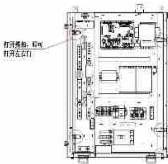
图 3-11 左右门搭扣开关位置图
