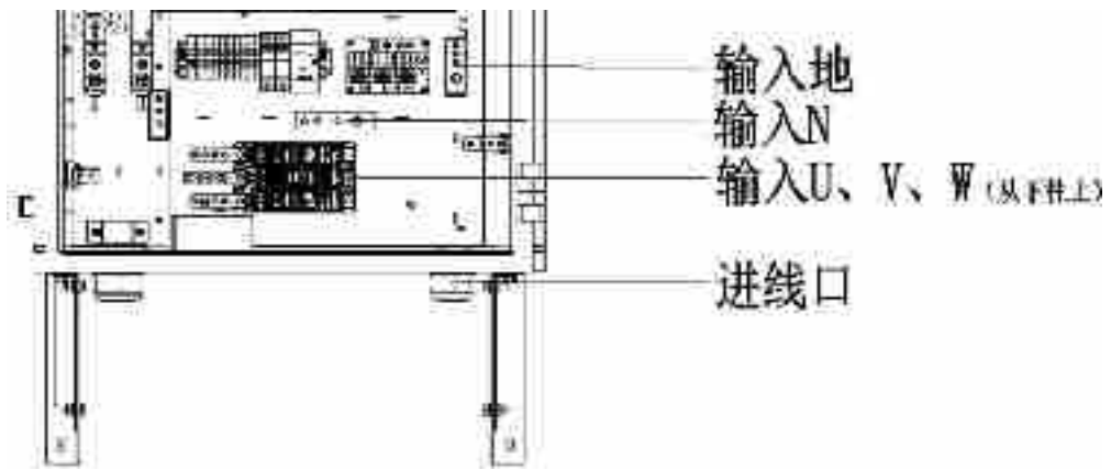
图 3-10 交流输入接线排示意图
