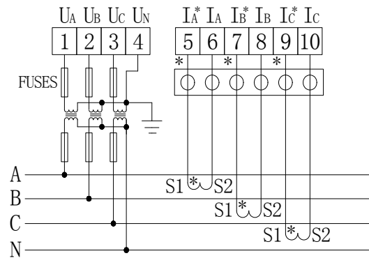
三相四线3PT、3CT
