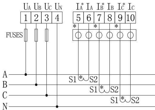
三相四线3CT
