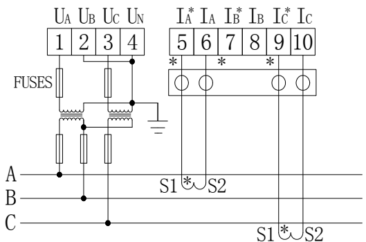
三相三线2PT、2CT
