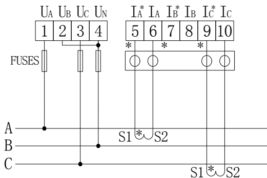
三相三线2CT
