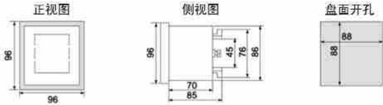
ACR220ELH 尺寸
