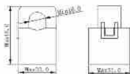
Φ 16mm
