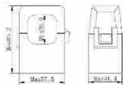
Φ 36mm
