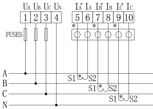
三相四线3CT
