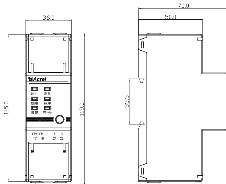
图 1 ARCM310
