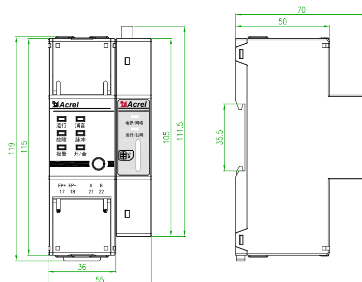
图 2 ARCM310-4G
